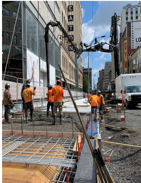
Bétonnage dalles trottoirs
